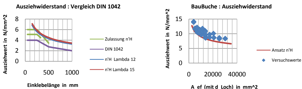
Abbildung 11: Ausziehwiiderstand in Funktion der Länge bzw. der Bruchfläche
